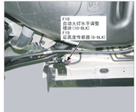
96. 后悬架左侧
